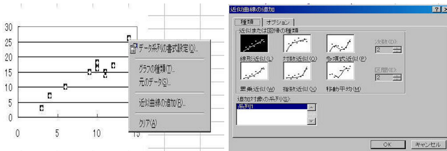
図 13 回帰直線
