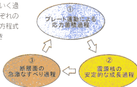
地震発生過程のサイクル
